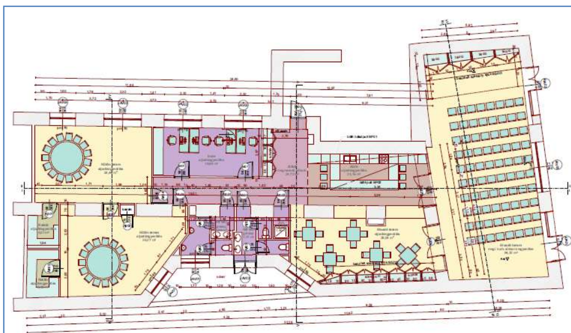
A Háló Közösségi és Kulturális Központ tervezett alaprajza
